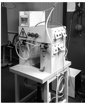
NMR装置
